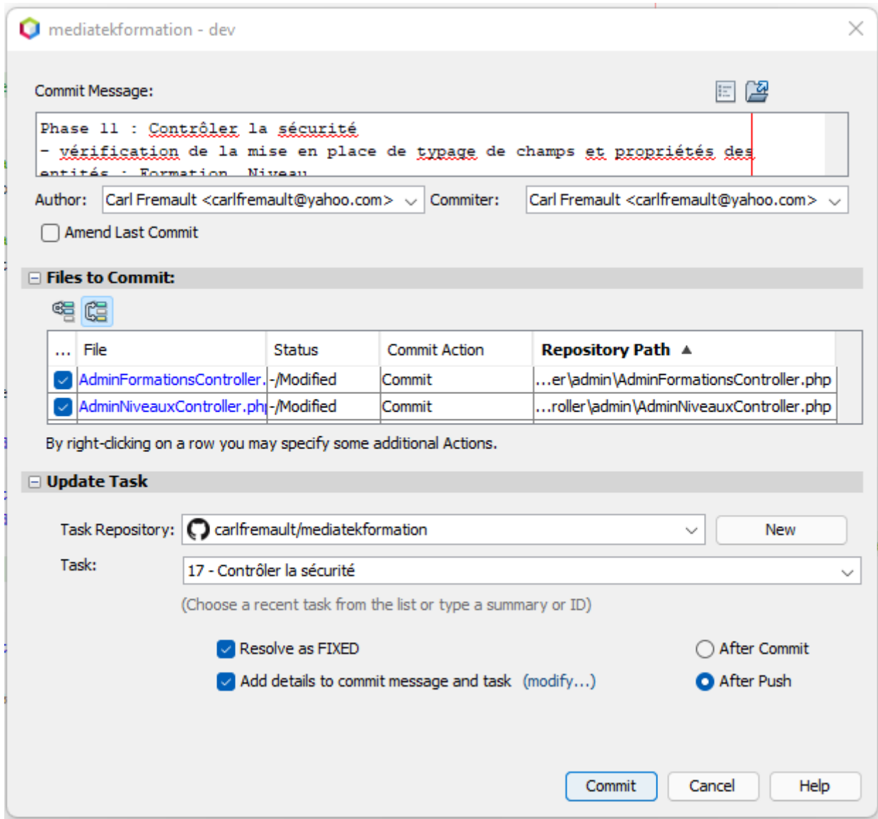
Figure 77: Commit avec mise à jour de tâche de suivi
