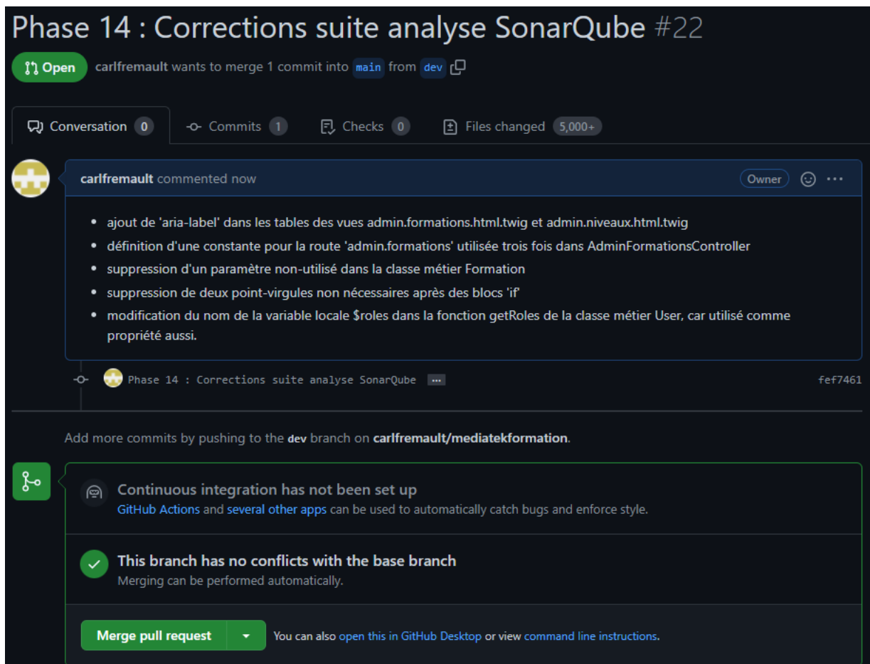
Figure 94: Commit après corrections
