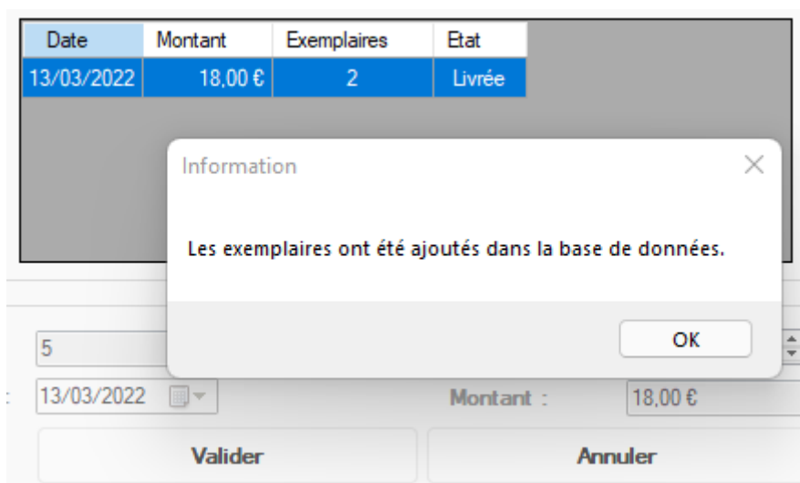
Figure 86: Confirmation d'ajout
